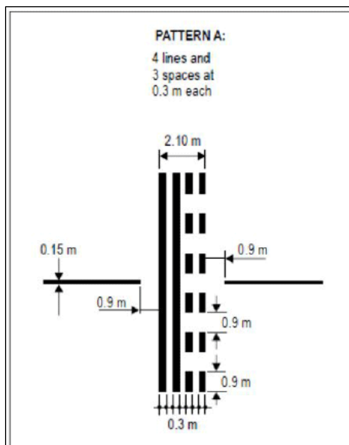
Figura 10 - Segnaletica orizzontale RHP
